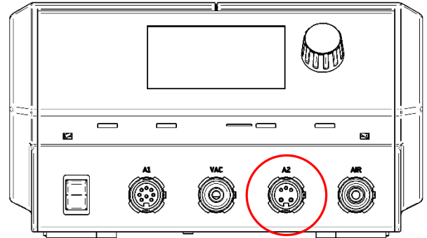
Abbildung / Figure 2: A2 Anschluss / socket i-CON VARIO 2
